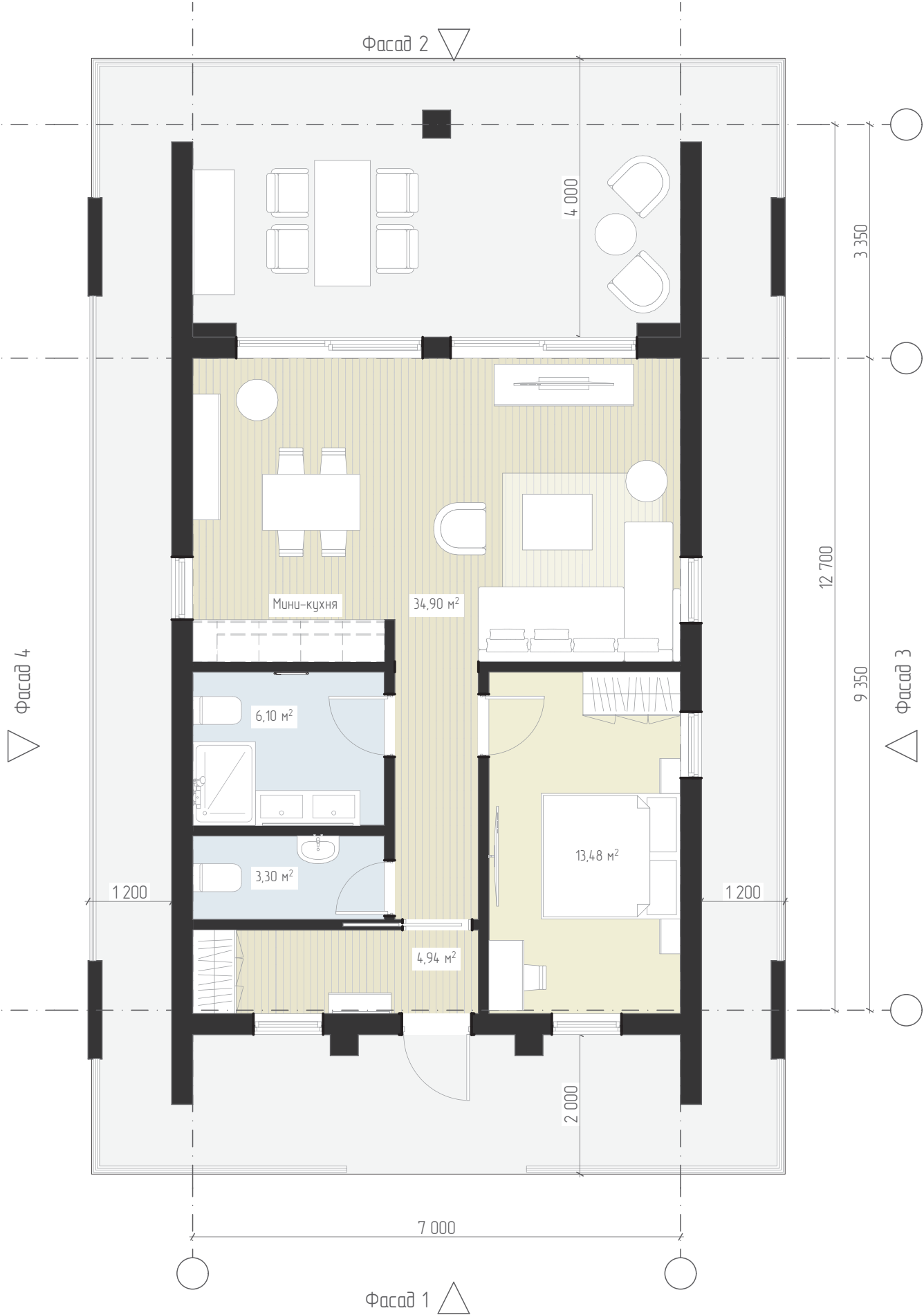
Планировочное решение вариант 2
