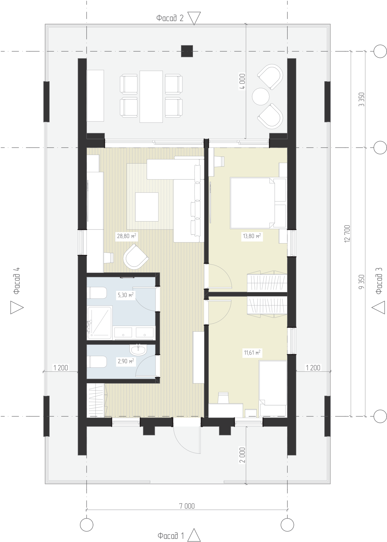
Планировочное решение вариант 1
